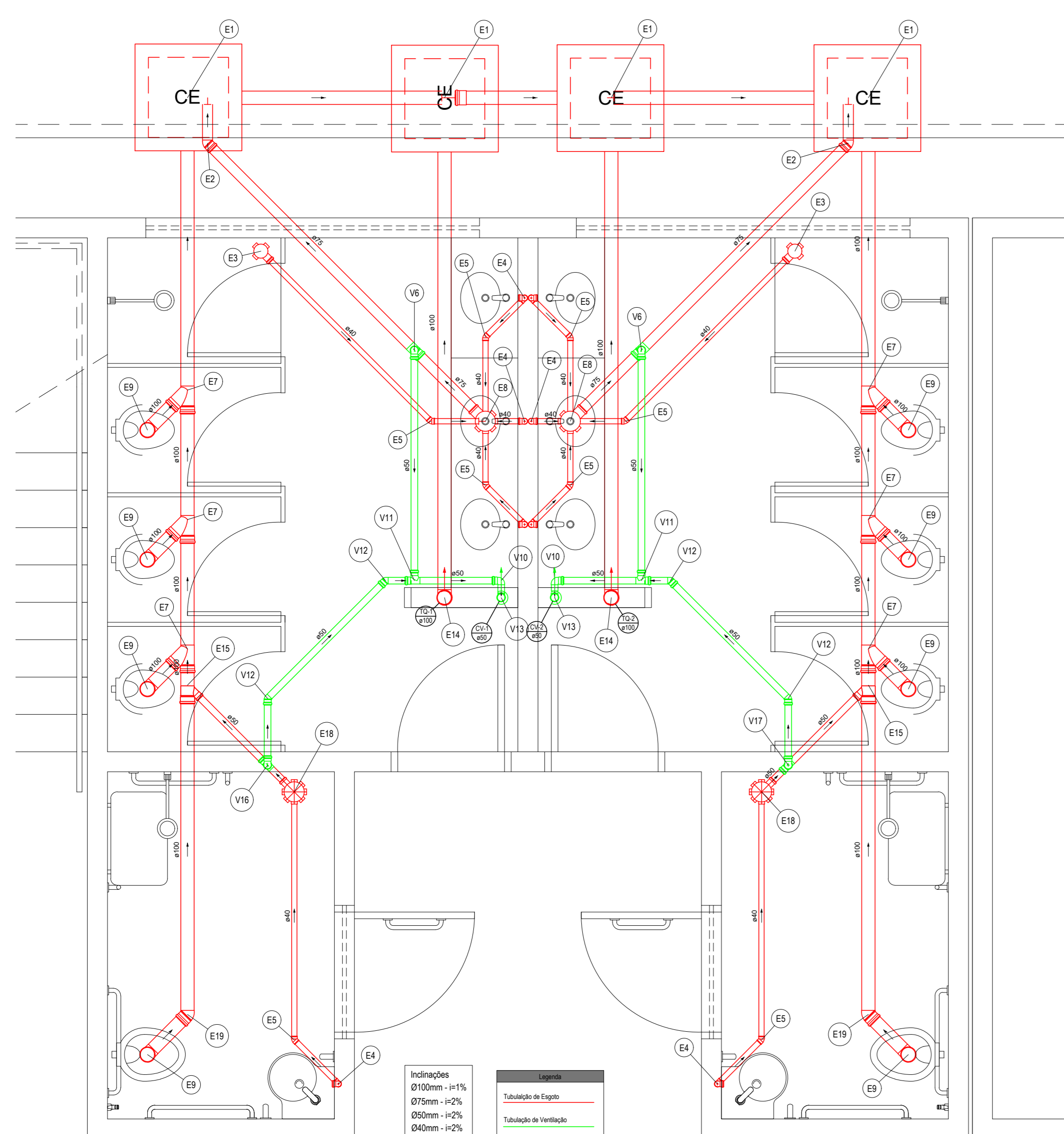
Detalhe S1 Escala 1:25
